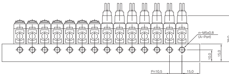
매니폴더 치수
