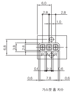
가스켓 홈 치수
