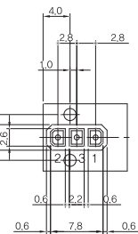
가스켓 홀 치수
