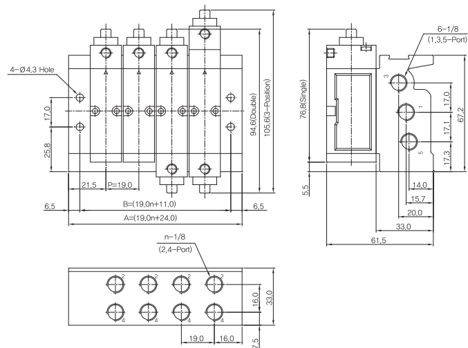
매니폴더 치수
