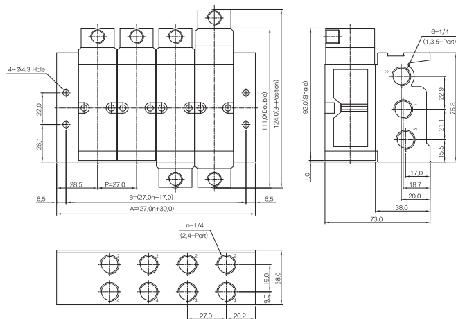
매니폴더 치수
