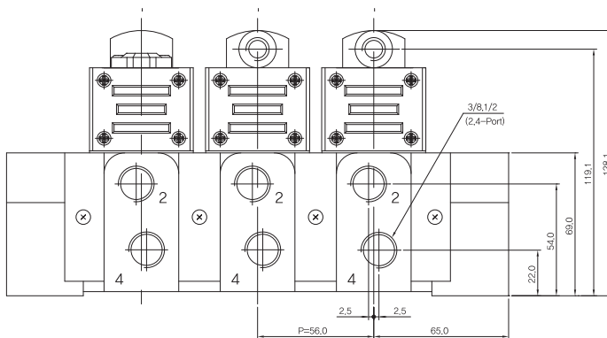
DOUBLE MANIFOLD BLOCK 치수
