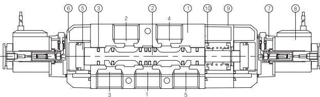
3위치 PAB Pressure Center(SF6503-IP-SD2-OO)
