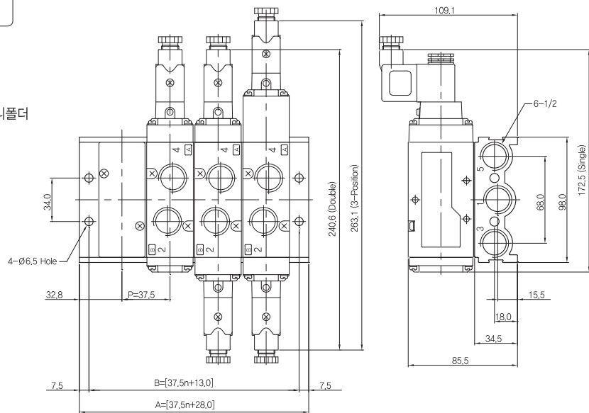
매니폴더 치수
