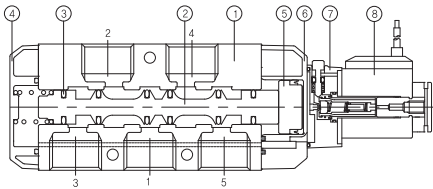
3위치 올포트블럭 Close Center(SF6303-IP-SD2-OO)
