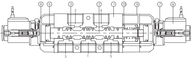
3위치 ABR Exhaust Center(SF6403-IP-SD2-OO)
