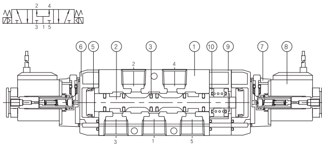
3위치 PAB Pressure Center(SF3503-IP-SD2-00)
