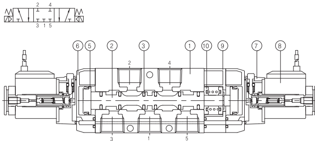
3위치 ABR Exhaust Center(SF5403-IP-SD2-00)
