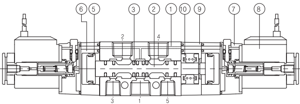
3위치 PAB Pressure Center(SF3503-IP-SD2-00)
