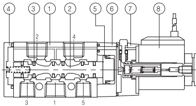
3위치 올포트블럭 Close Center(SF4303-IP-SD2-00)
