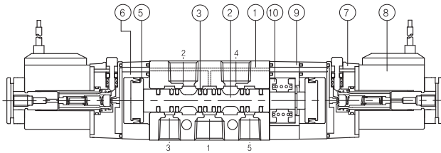
3위치 ABR Exhaust Center(SF4403-IP-SD2-00)
