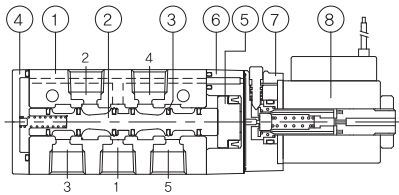
3위치 오픈포트블럭 Close Center(SF2303-IP-SD1-OO)
