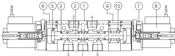
3위치 PAB Pressure Center(SF2503-IP-SD1-OO)
