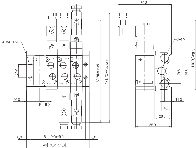
매니폴더 치수
