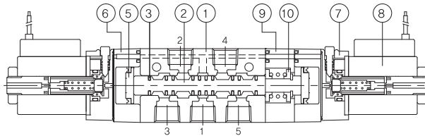
3위치 ABR Exhaust Center(SF2403-IP-SD1-OO)
