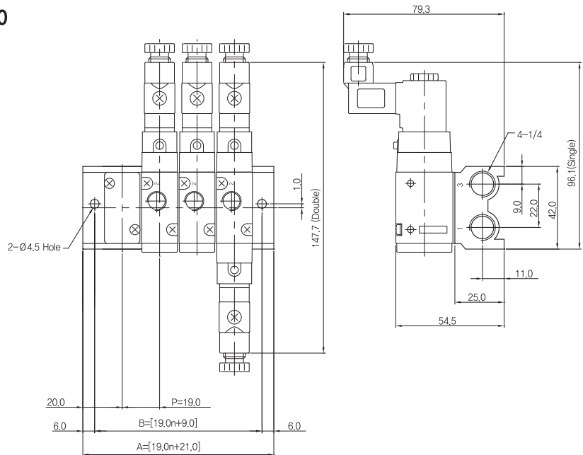
매니폴더 치수
