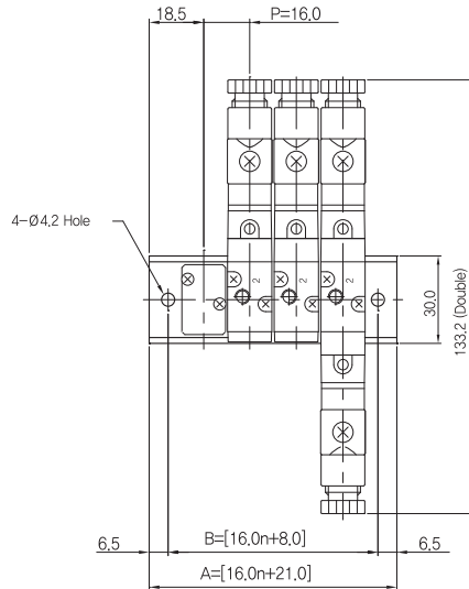
매니폴더 치수
