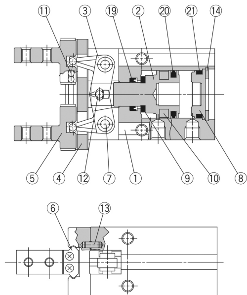
Greifer geschlossen
