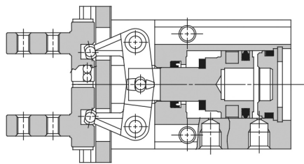
Greifer geschlossen
