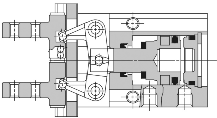
Greifer geschlossen
