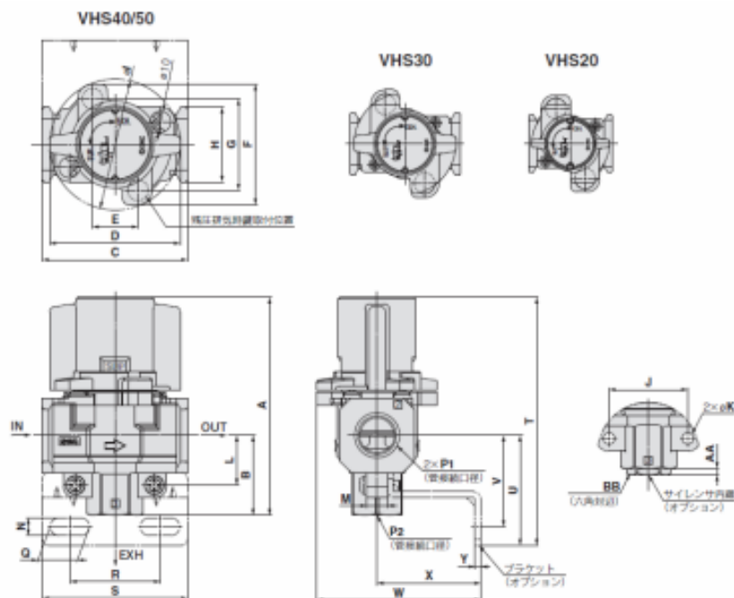
外形寸法
