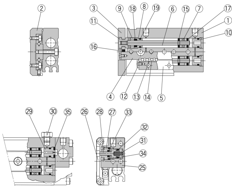
Mit Endlagenverriegelung
