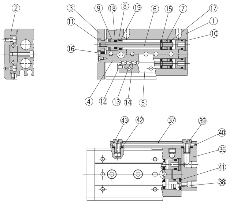
Axialer Luftanschluss
