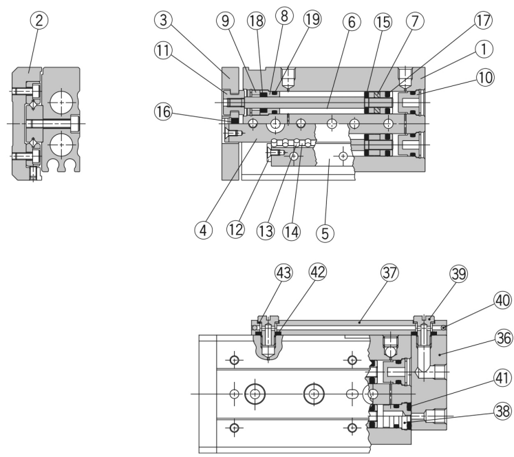
Axialer Luftanschluss
