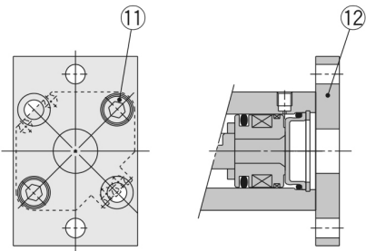
Flansch hinten (G)
