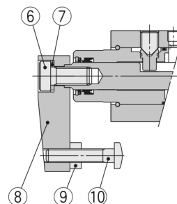
Flansch hinten (G)
