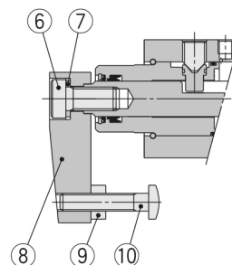
Flansch hinten (G)
