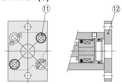
Flansch hinten (G)
