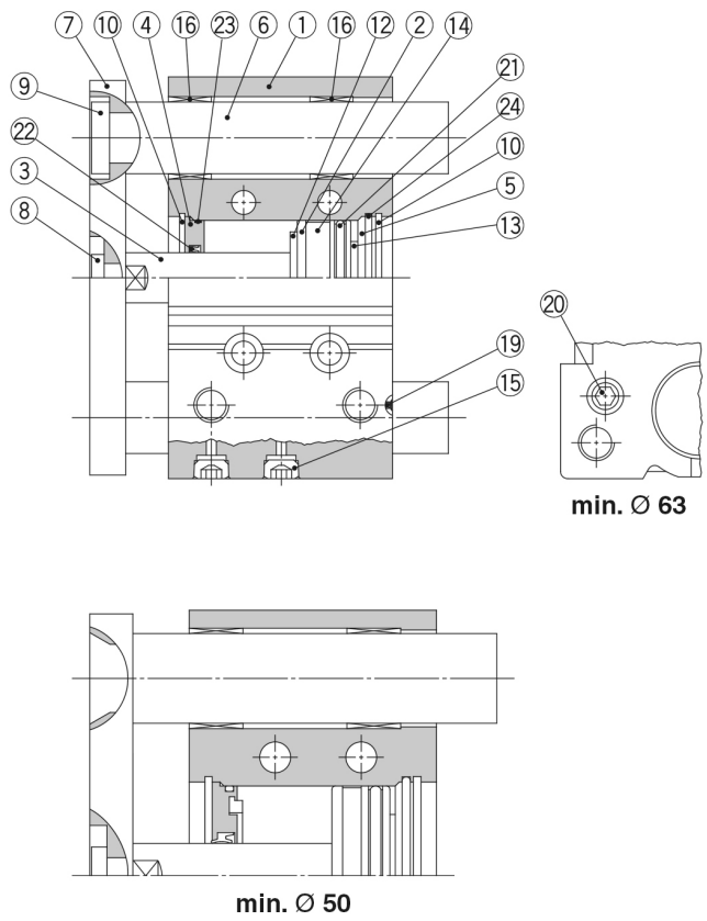
min. Ø 50
