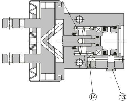
Drucklos geschlossen
