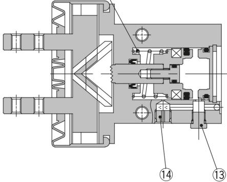
Drucklos geschlossen
