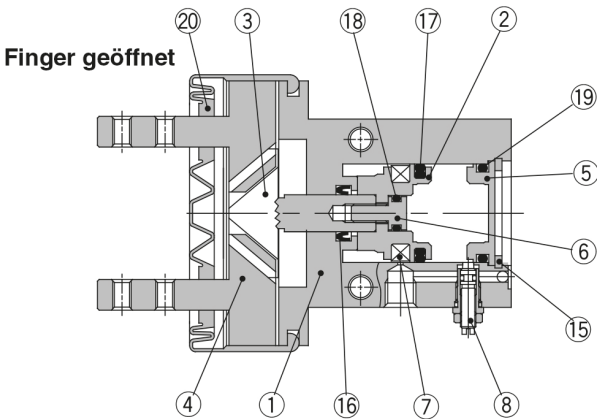
Doppeltwirkend
