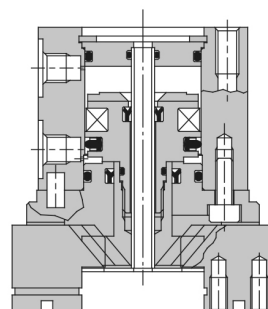
Ø32 bis Ø80 Finger geöffnet
