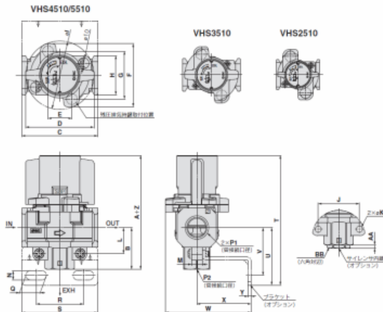
外形寸法図
