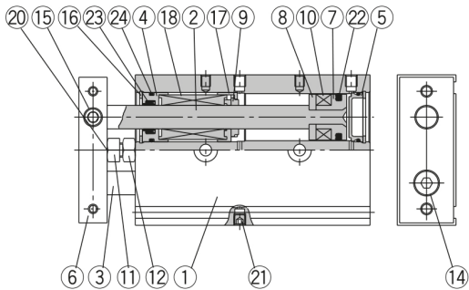
CXSL20 bis 32
