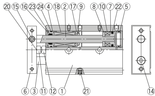
CXSL20 bis 32
