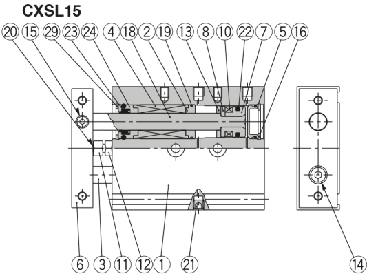
Stückliste: Standard-Luftanschluss
