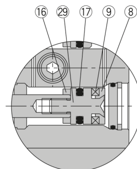
Tige du piston B
