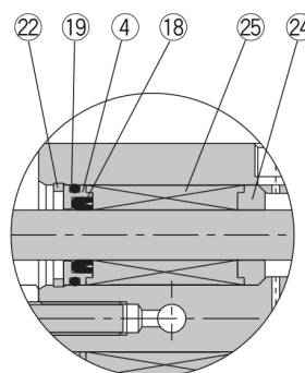
Zylinderkopf
