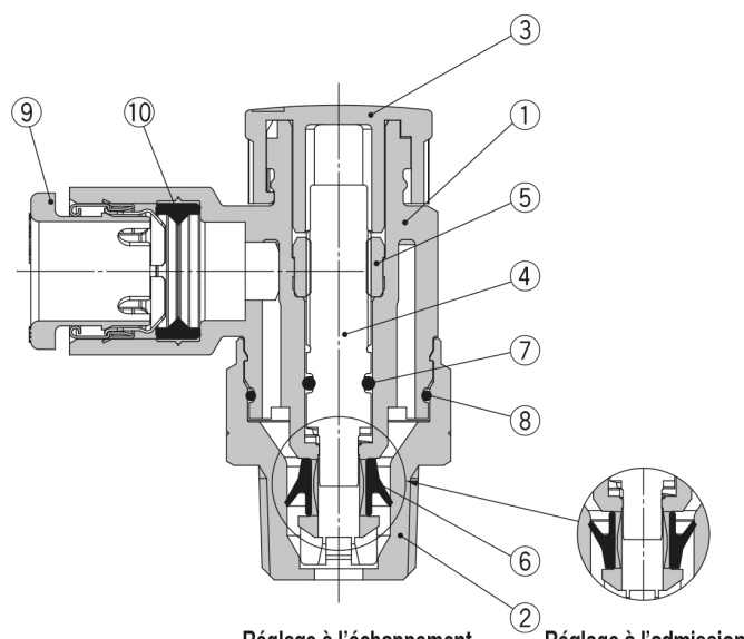
Nomenclature Réglage à l'échappement Réglage à l'admission
