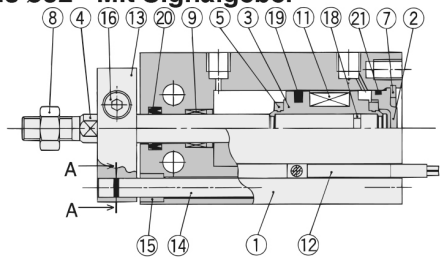
ø16 bis ø32 Mit Signalgeber
