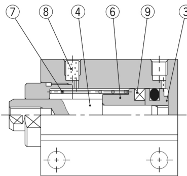
eingebauter Magnetring
