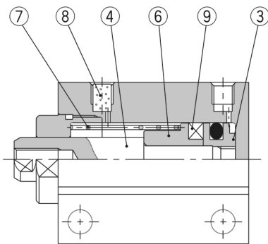
eingebauter Magnetring
