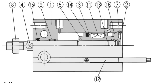
ø16 bis ø32 Mit Signalgeber
