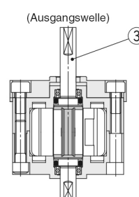
Durchgehende Welle
