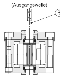
Durchgehende Welle
