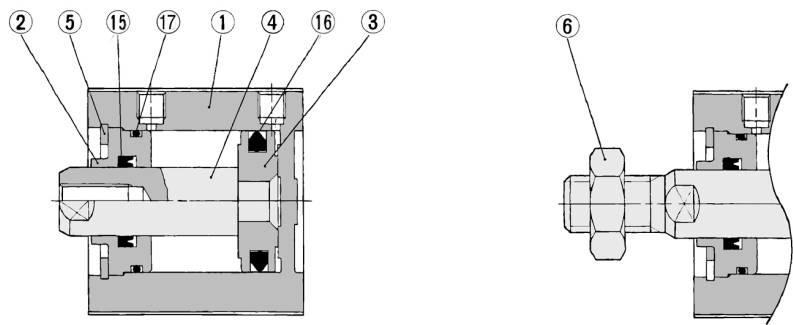
Tige taraudée
