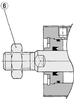
Kolbenstangen- Außengewinde
