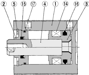
Mit Signalgeber (eingebauter Magnetring) ø20, ø25
