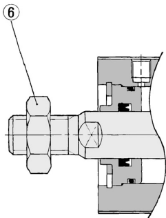
Kolbenstangen- Außengewinde
