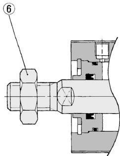
Kolbenstangen- Außengewinde
