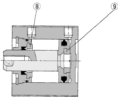
Mit elastischen Dämpfscheiben
