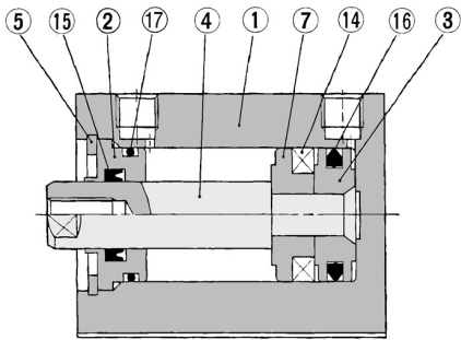
Mit Signalgeber (eingebauter Magnetring) ø12, ø16
