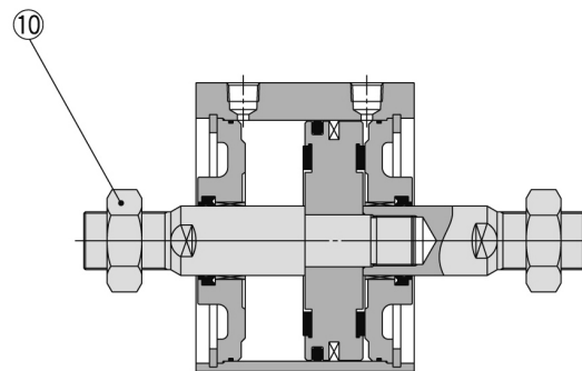
Kolbenstangen-Außengewinde
