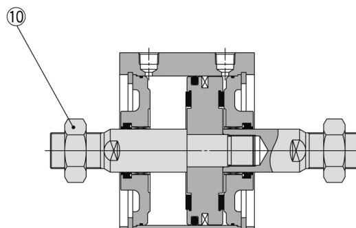
Kolbenstangen-Außengewinde
