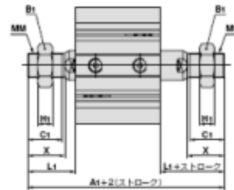
ロッド先端おねじ
