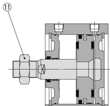
Kolbenstangen-Außengewinde
