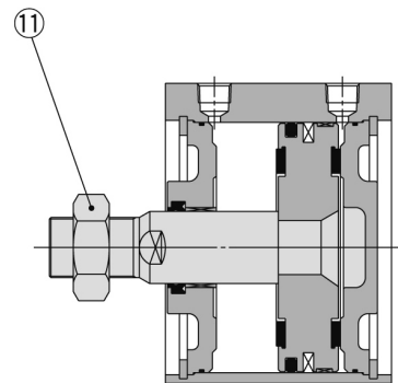
Kolbenstangen-Außengewinde
