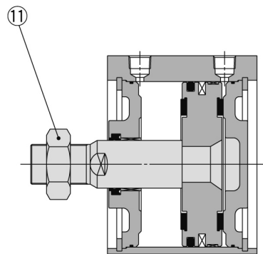
Kolbenstangen-Außengewinde
