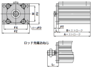
ロッド側フランジ形/CDQ2F
